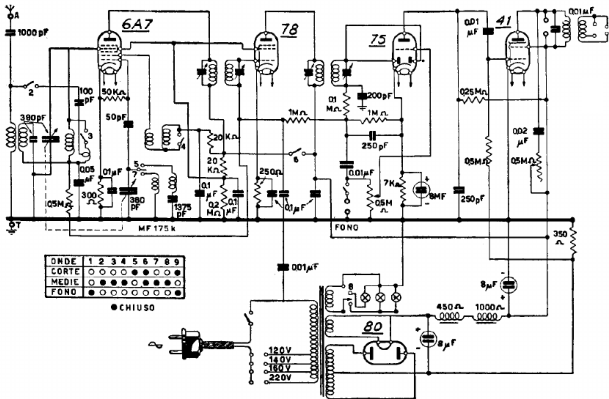
WATT RADIO. — Mod. « Ondina Vª e Sirena ». — Media frequenza: 175 kHz. — Gamme: corte e medie. — Produzione 1936-1937
